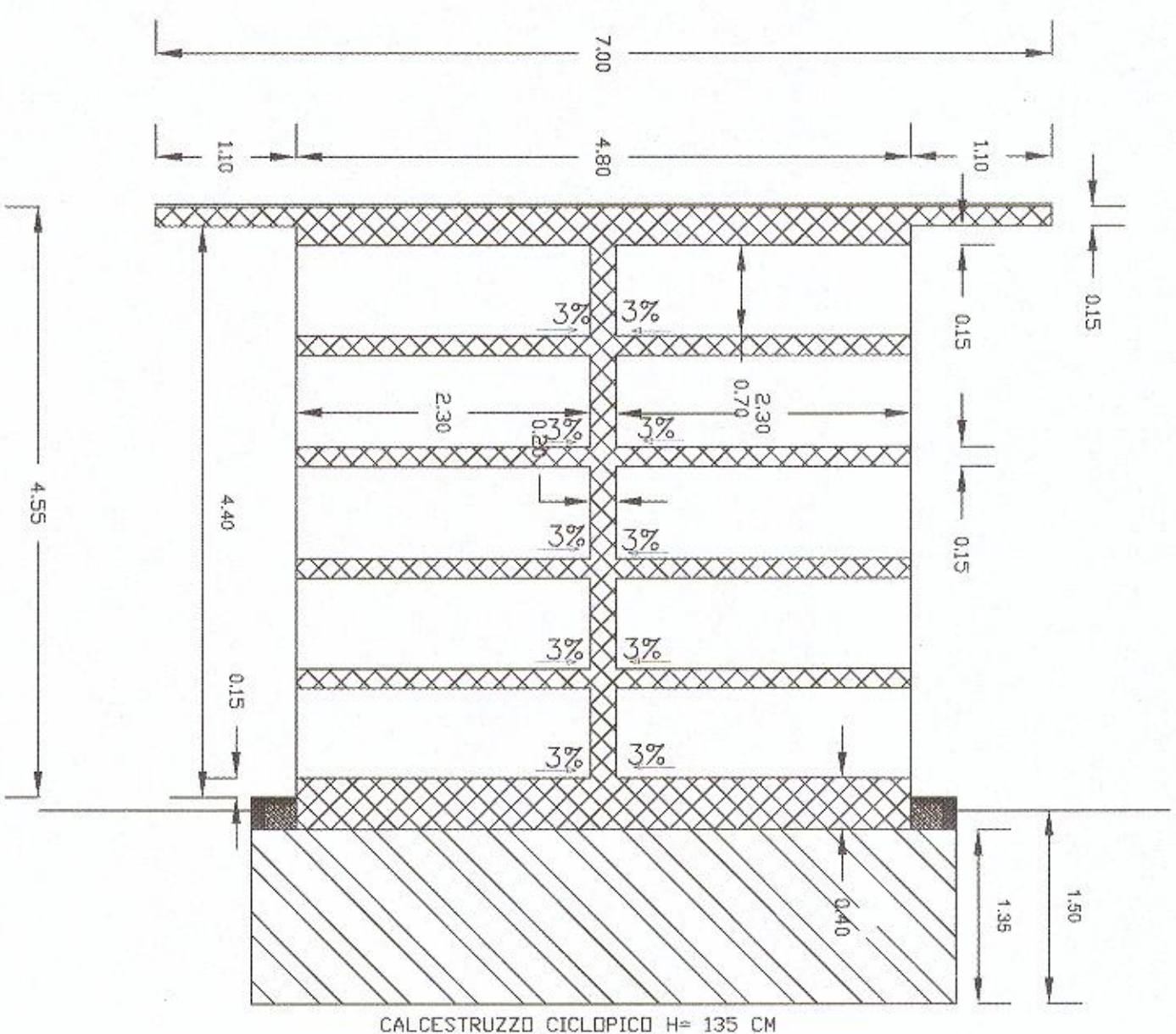
SEZIONE A-A
