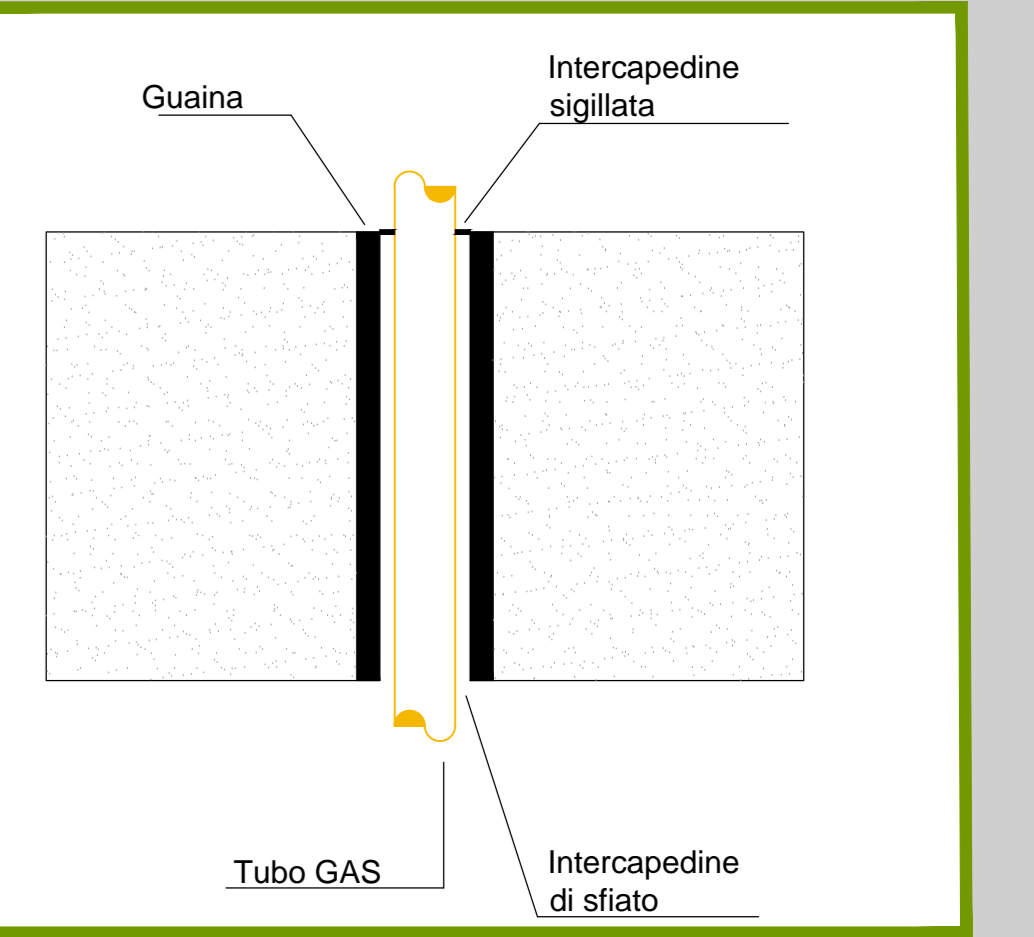
ATTRAVERSAMENTI PARETI E SOLAI DELLE TUBAZIONI
