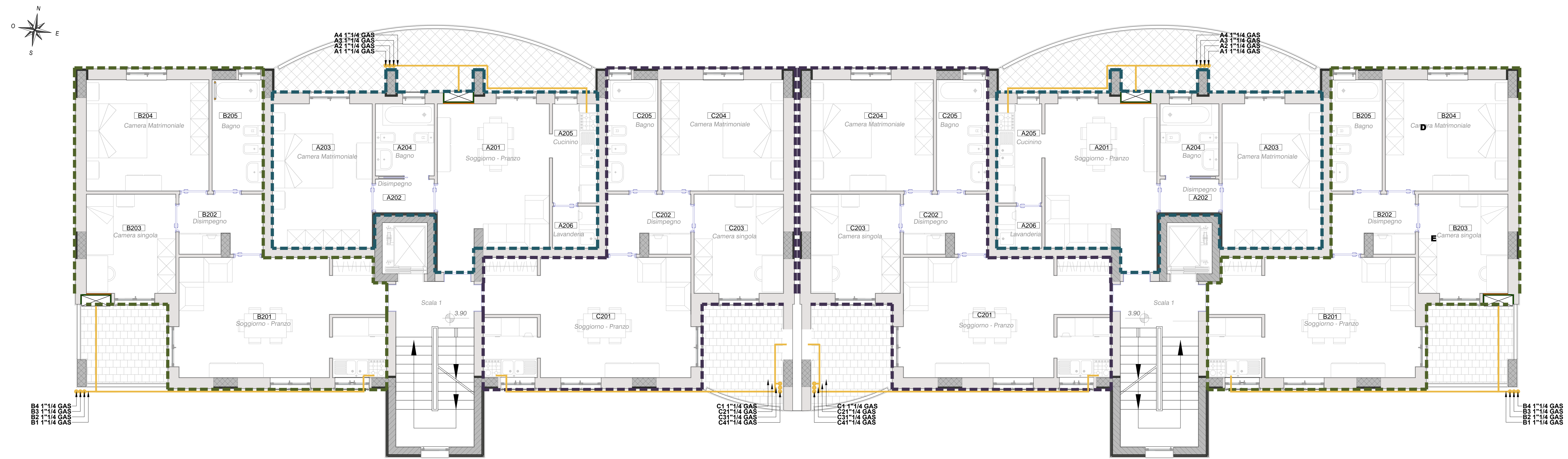
PIANTA PIANO PRIMO
