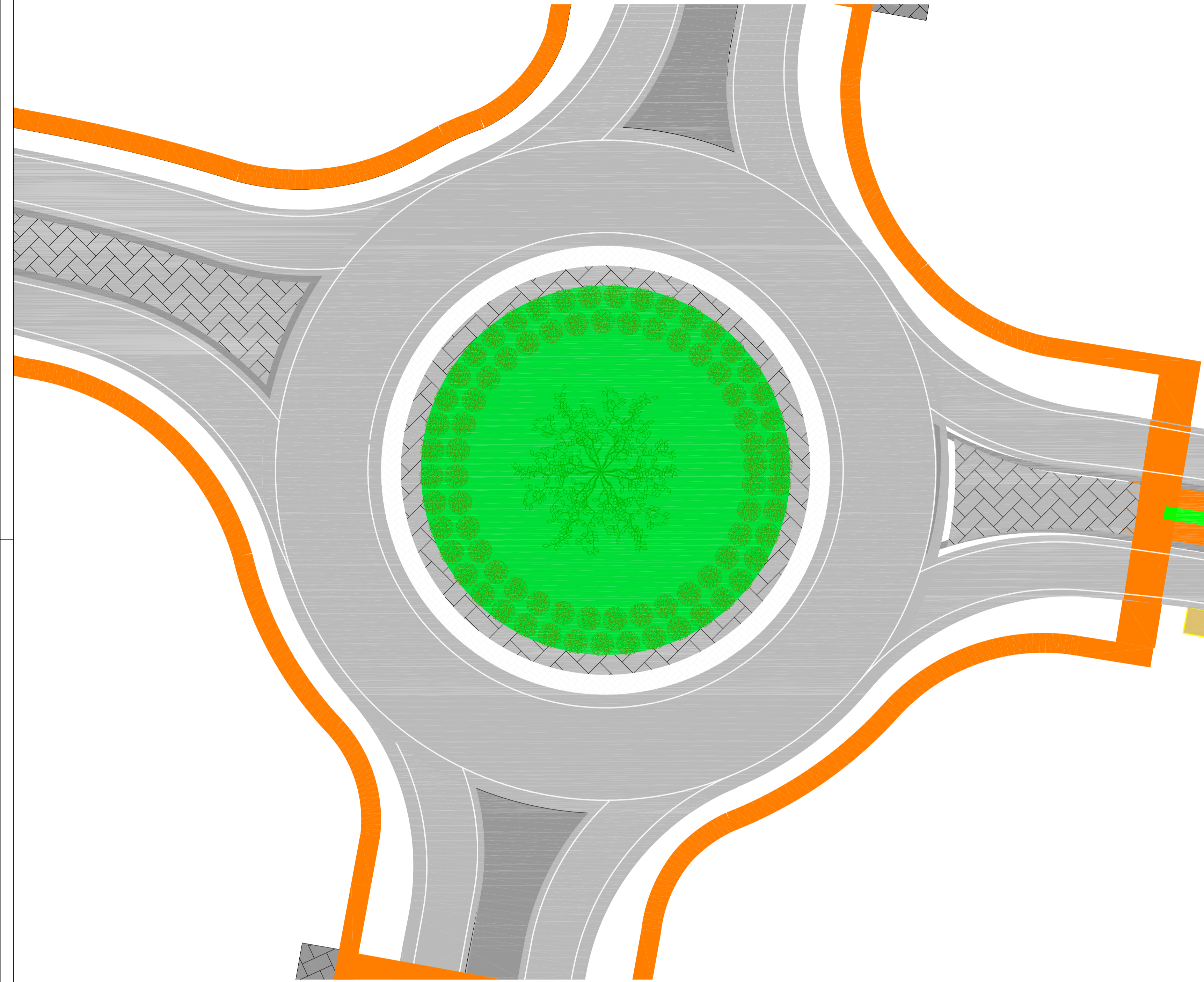
PLANIMETRIA Scala 1:200
