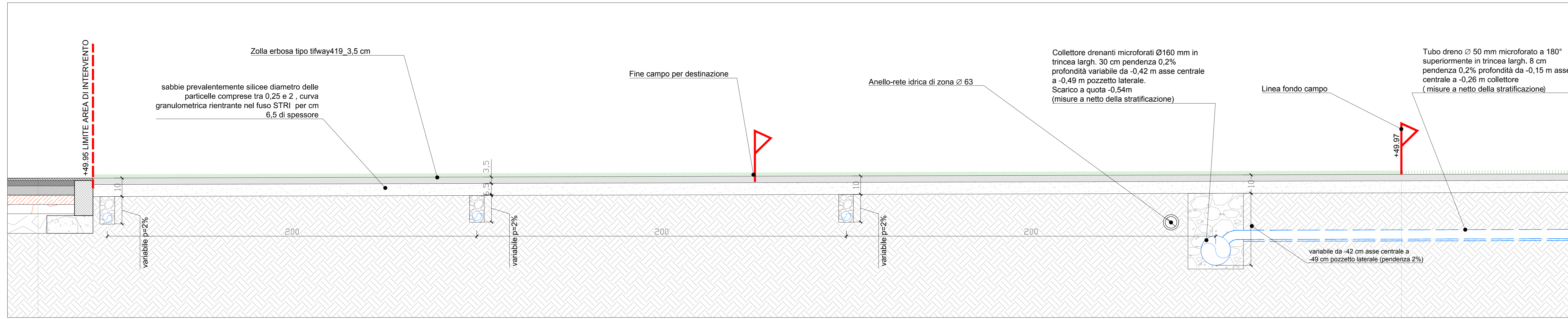
SEZIONE LONGITUDINALE (C)
