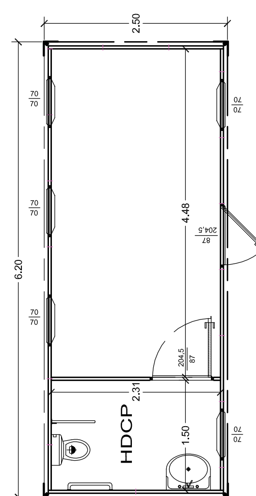
Partic. A - POSTO PRONTO SOCCORSO - N.1 MODULO - Scala 1:50
