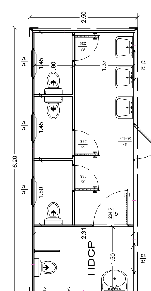
Partic. C - SERVIZI IGIENICI DONNE - N.1 MODULO - Scala 1:50
