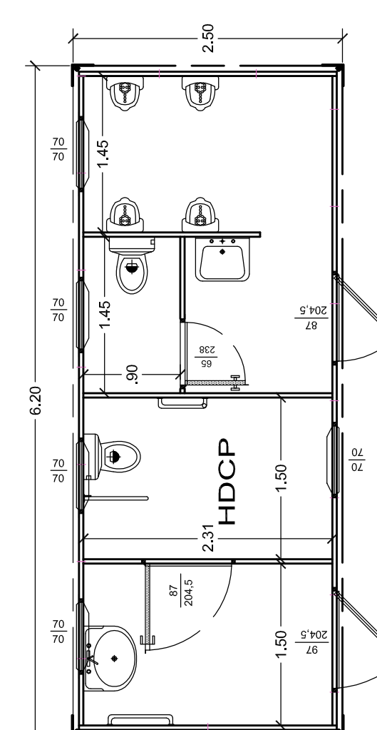
Partic. B - SERVIZI IGIENICI UOMINI - N.2 MODULI - Scala 1:50
