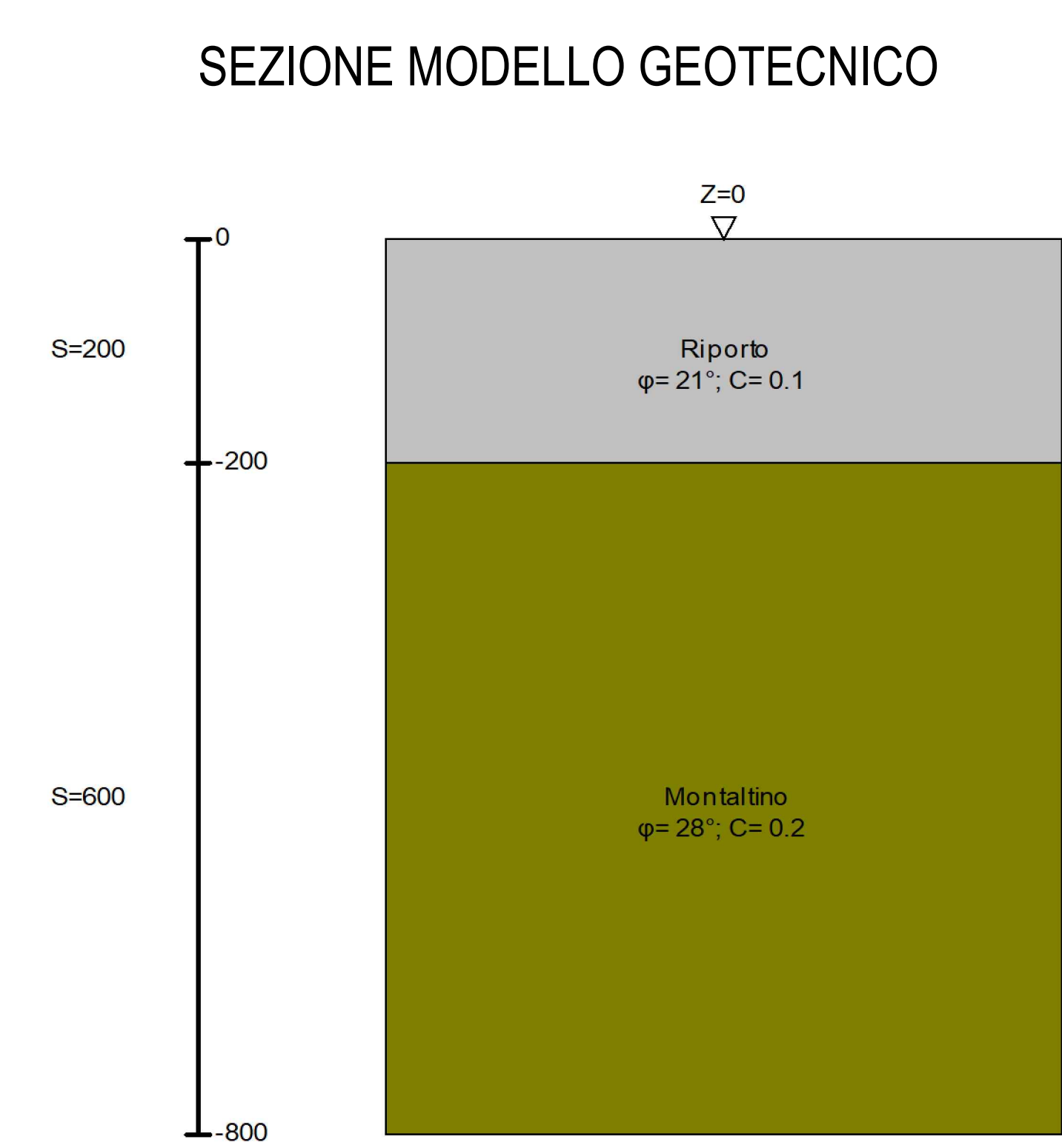
INDAGINI GEOTECNICHE AREA IMPIANTO IS1 - scala 1:200
