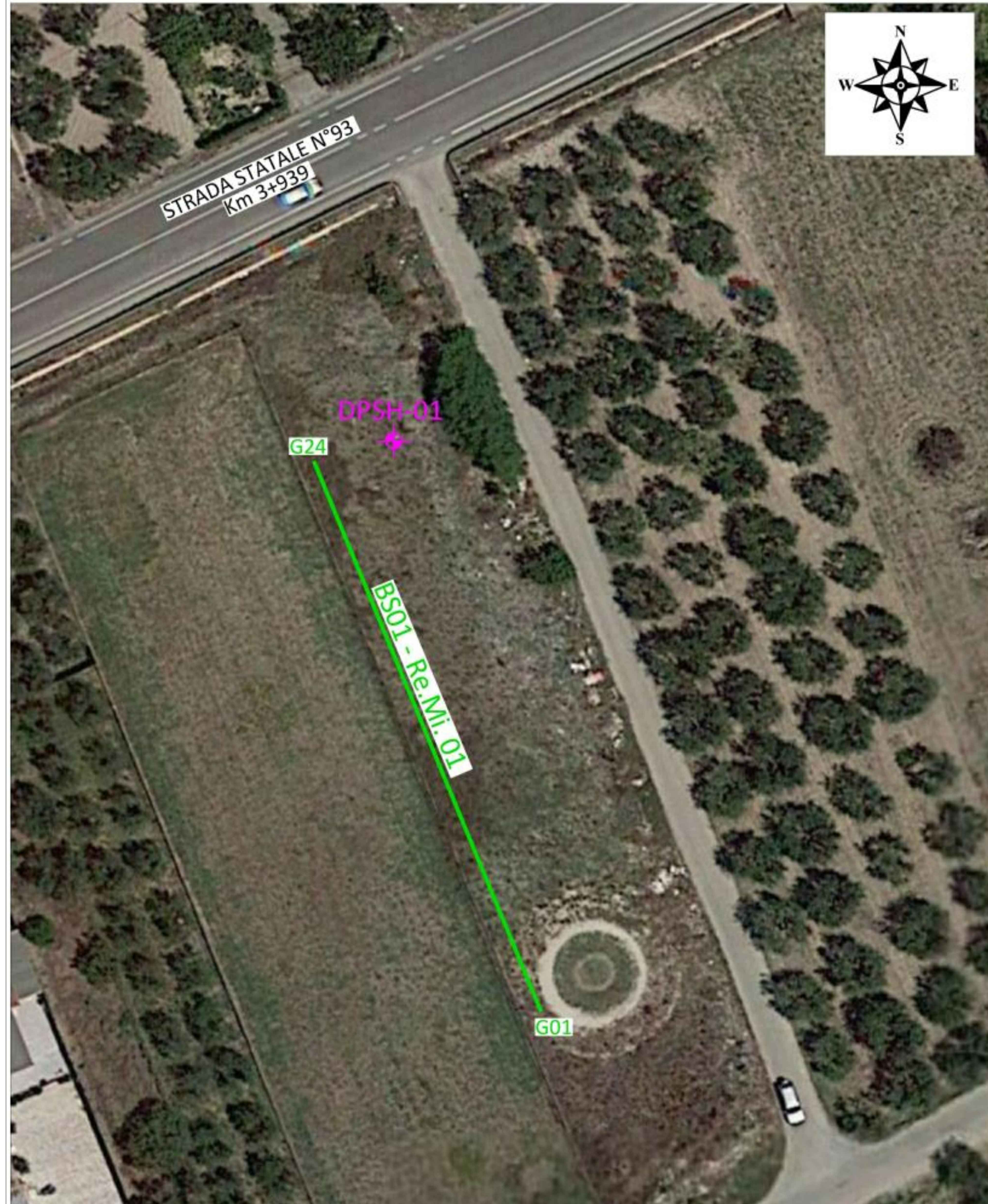
INDAGINI GEOTECNICHE AREA IMPIANTO IS1 - scala 1:200
