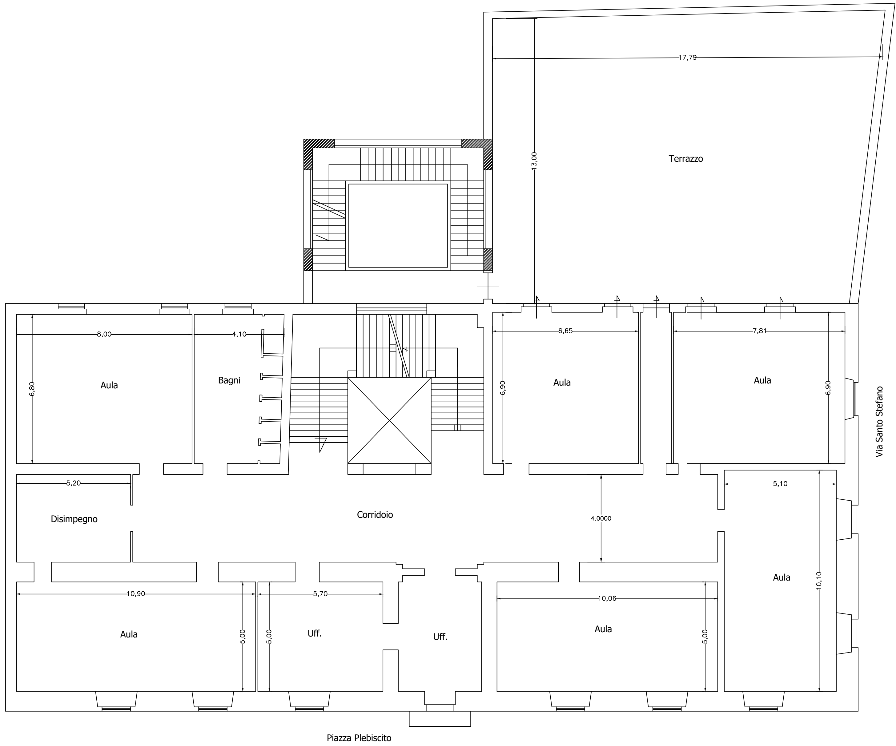
PLANIMETRIA PRIMO PIANO
