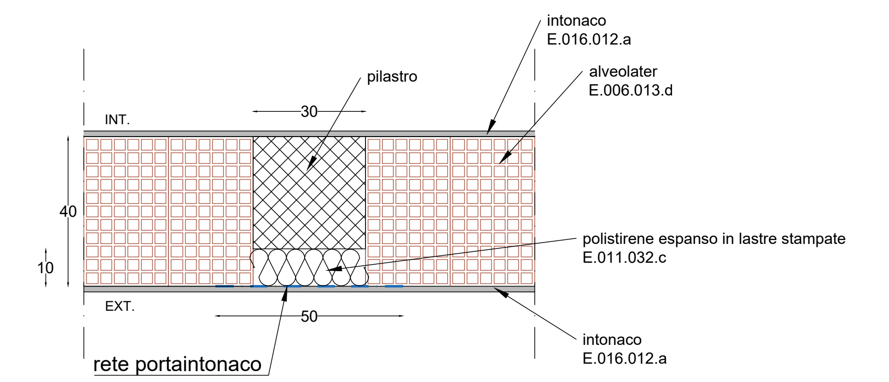
SEZIONE ORIZZONTALE MURO DI TOMPAGNO
