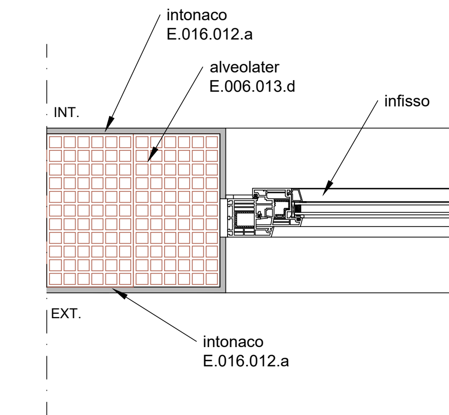
SEZIONE ORIZZONTALE ANCORAGGIO INFISSO
