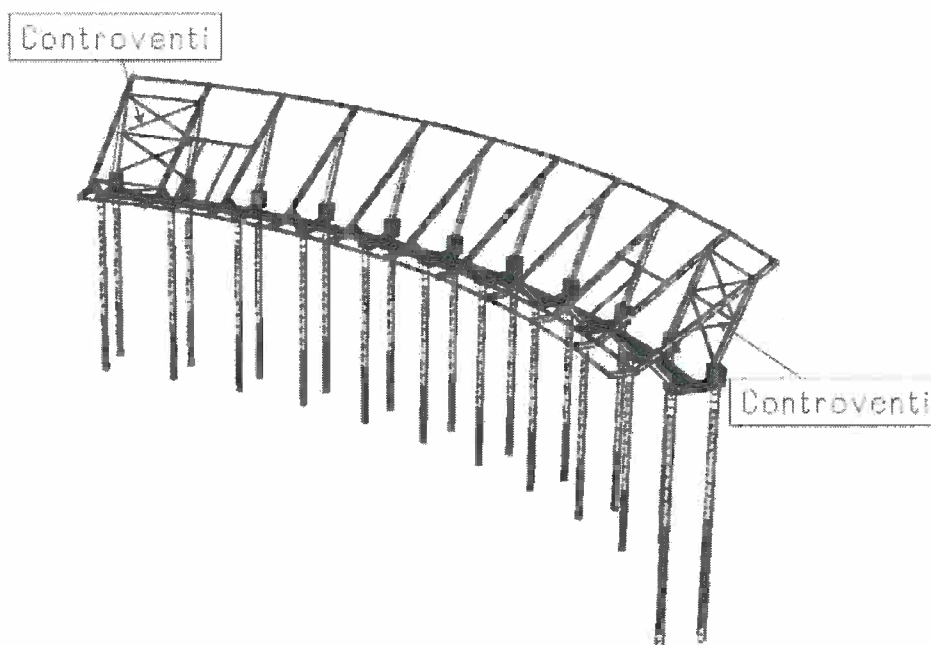
Figura 1 Modello Strutturale, vista controventi.
