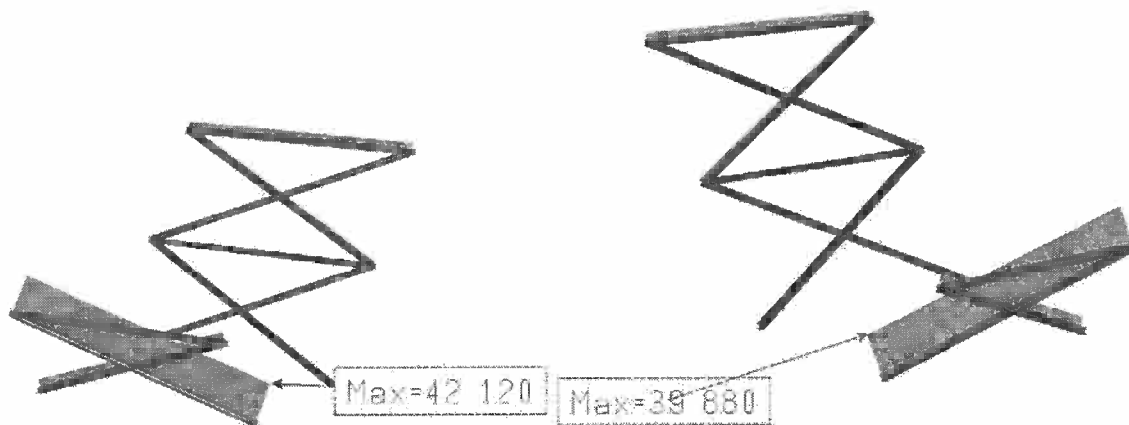
Figura 3 Sforzo normale nei Controventi.
