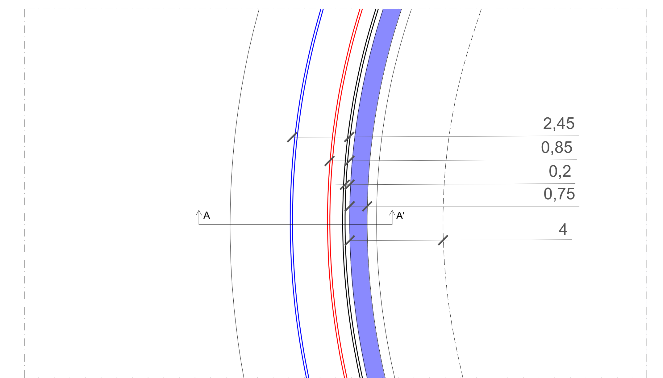
DETTAGLIO TRATTO CURVO 1:100
