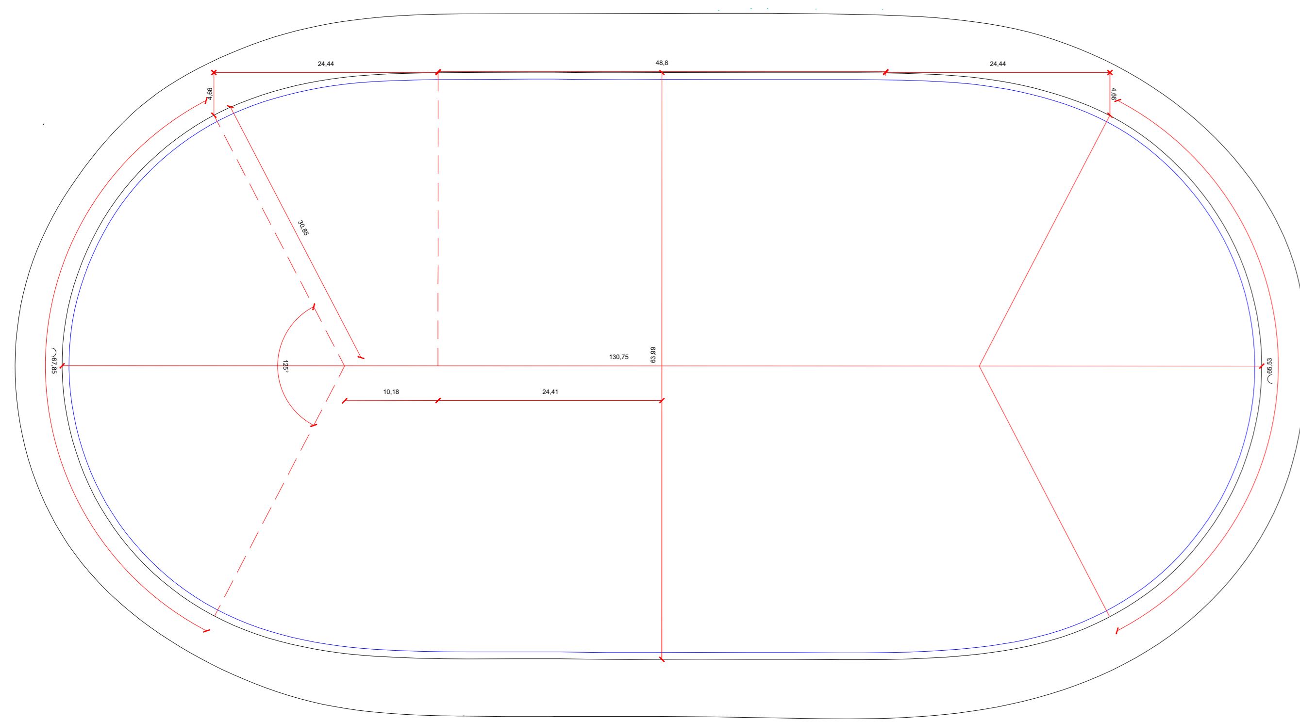
SVILUPPO GEOMETRICO PISTA 1:400
