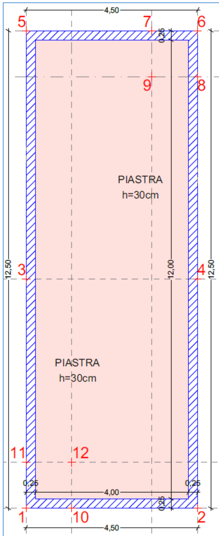
Pianta
