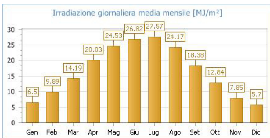
Fig. 1: Irradiazione giornaliera media mensile sul piano orizzontale [MJ/m 2 ]- Fonte dati: UNI 10349 - Località di riferimento: FOGGIA (FG)/BARI (BA)
