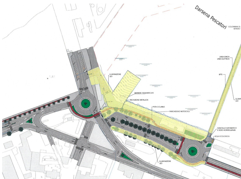
Figura 1 – Planimetria di progetto
